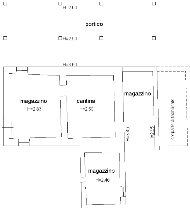
PIANO 1^ SOTTOSTRADA
